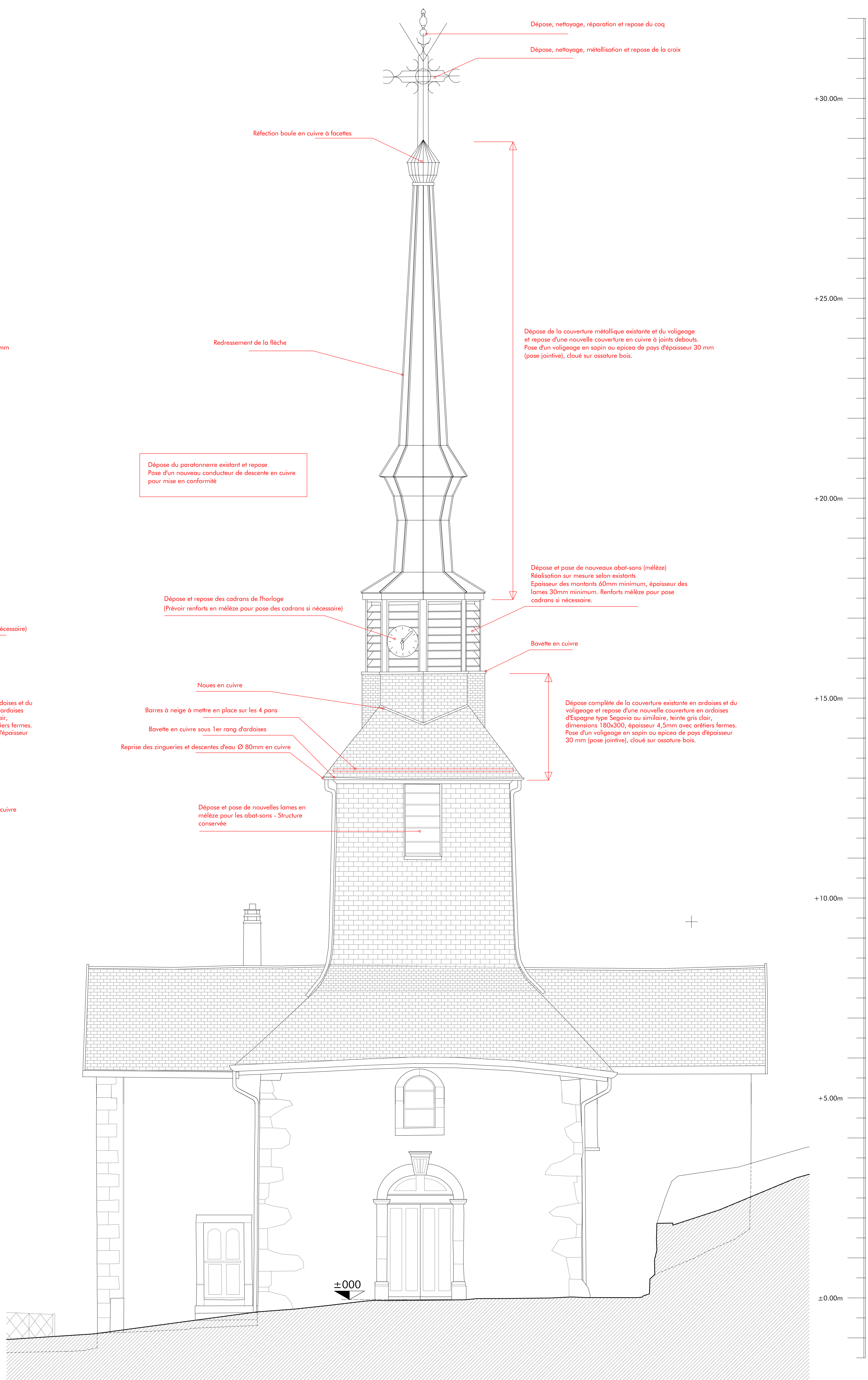
PROJET - FACADE OUEST
