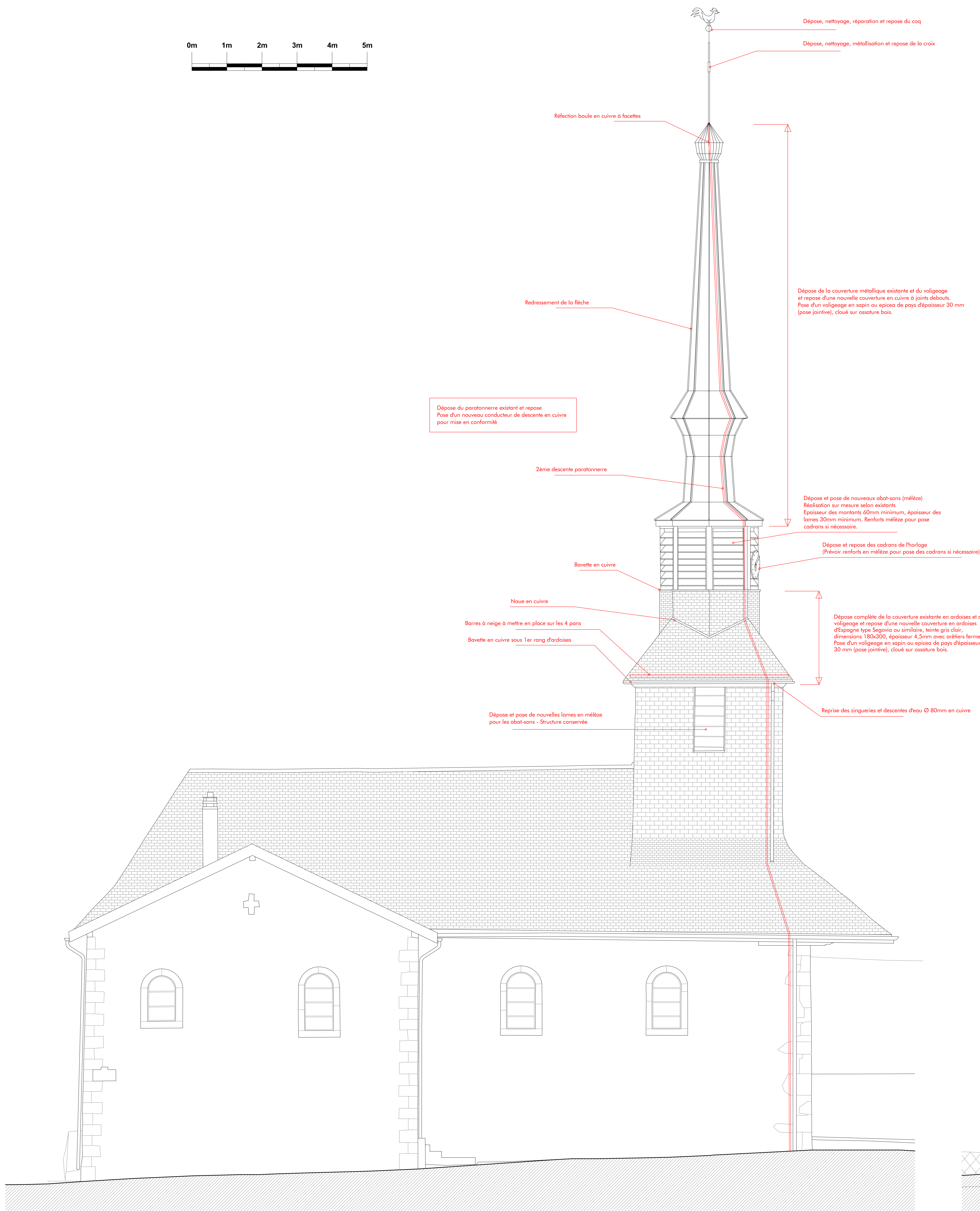
PROJET - FACADE NORD
